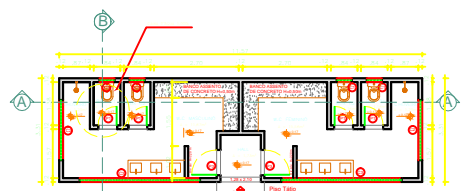
PLANTA BAIXA - W.C.
