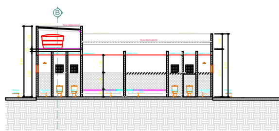
CORTE A-A'
