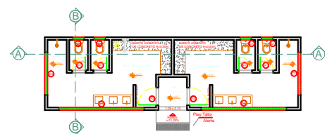
PLANTA BAIXA - LAYOUT W.C.
